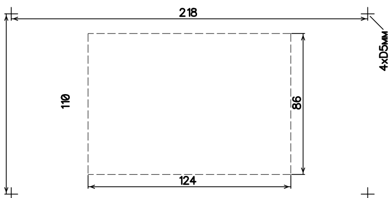
Рис. 3. Vario 3A24V с радиатором BPO1908
