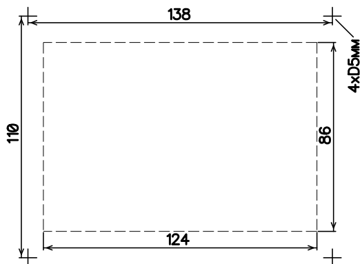
Рис. 1. Vario 2A24V с радиатором BPO1908
