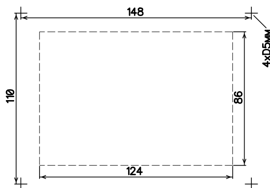
Рис. 4. Vario 3A24V с радиатором BPO1909
