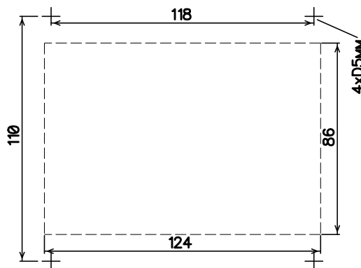
Рис. 2. Vario 2A24V с радиатором BPO1909
