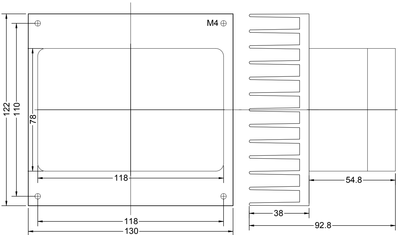
Vario 2A24V с радиатором БПО-1909
