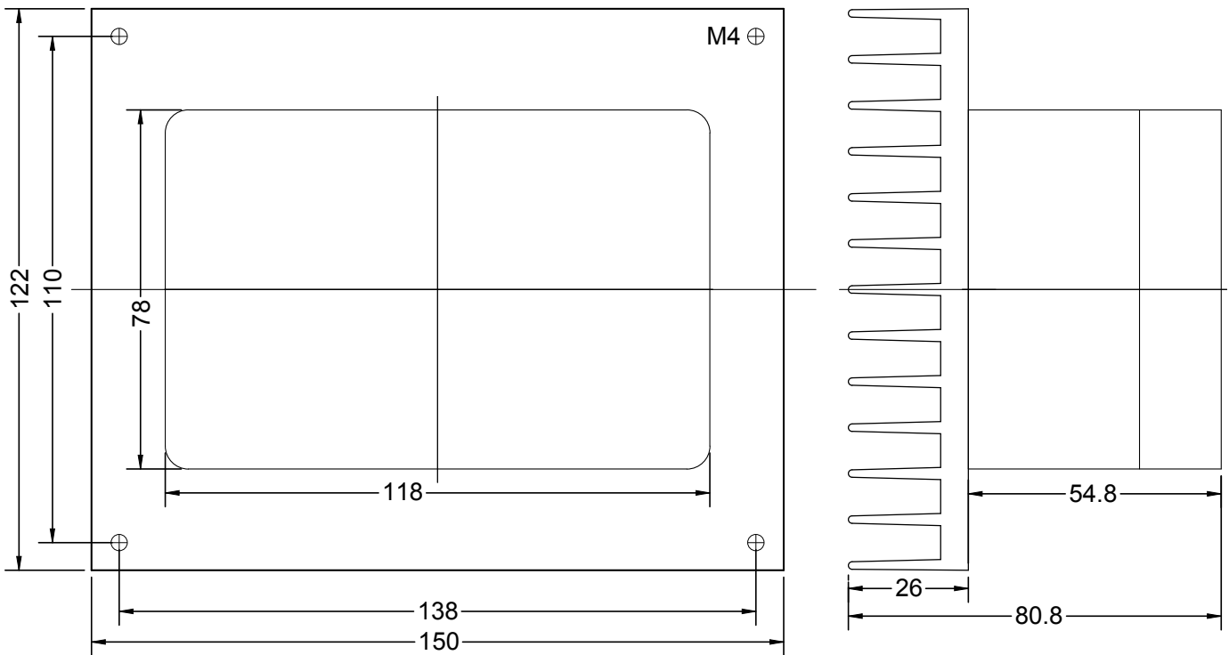
Vario 2A24V с радиатором БПО-1908
