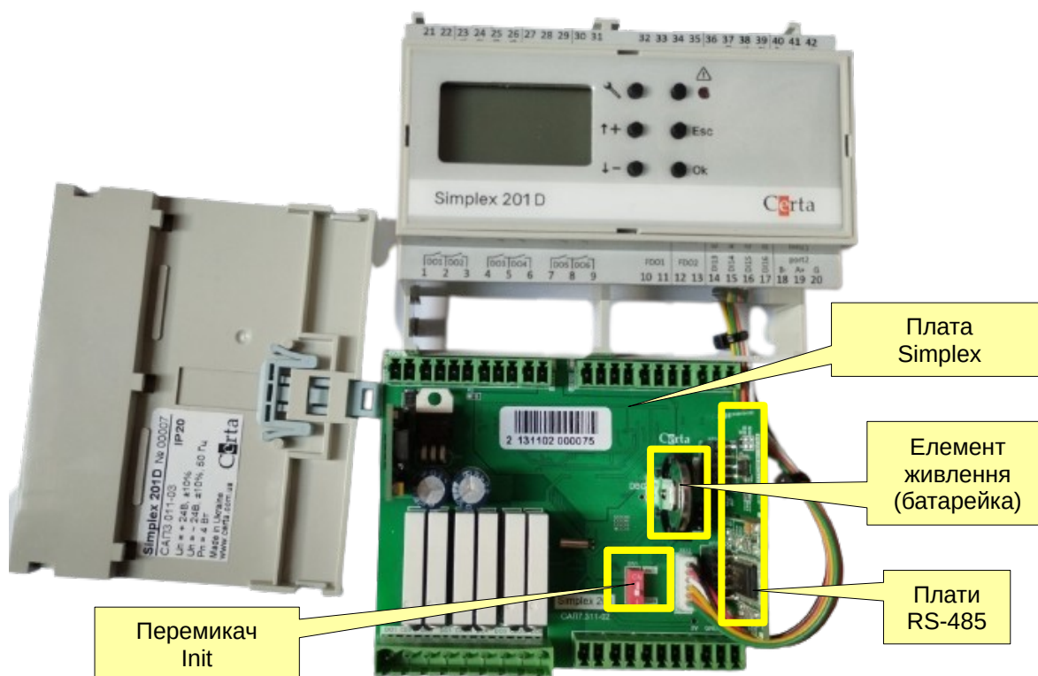
Рисунок 6 -Розібраний контролер
