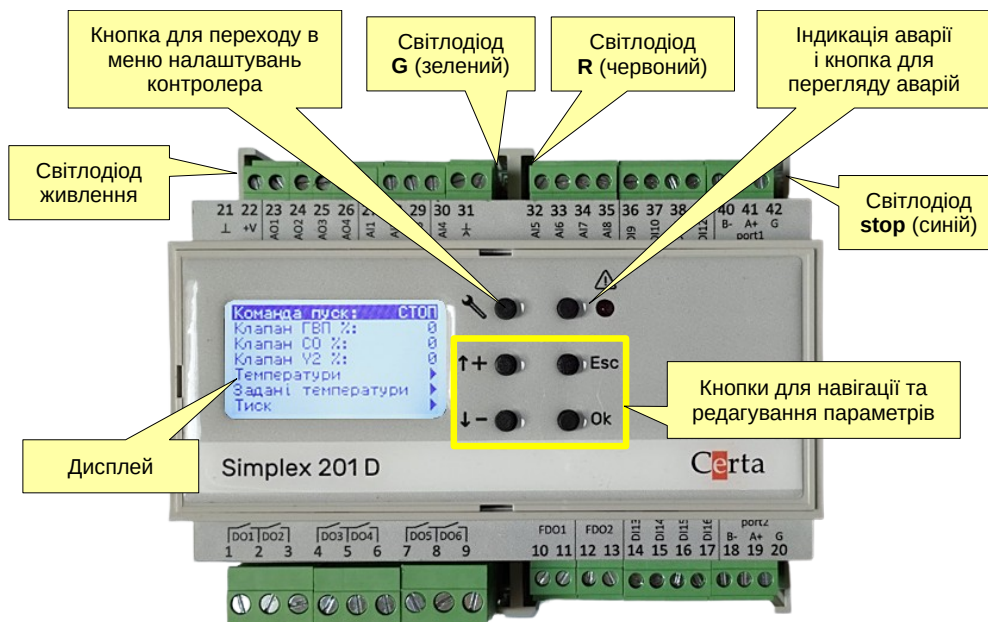
Рисунок 1 – Зовнішня будова Simplex 201D
