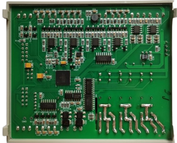
Рисунок 7 – Плата Simplex вставлена в корпус
