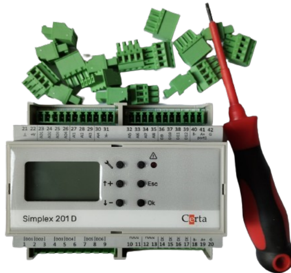
Рисунок 4 – Зняті клеми
