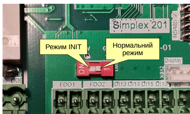
Рисунок 13 – Перемикач INIT
