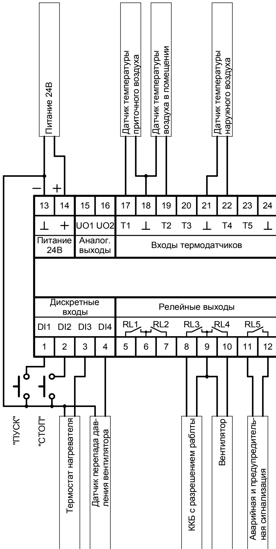
Рисунок 10. Подключение ККБ с разрешением работы.
