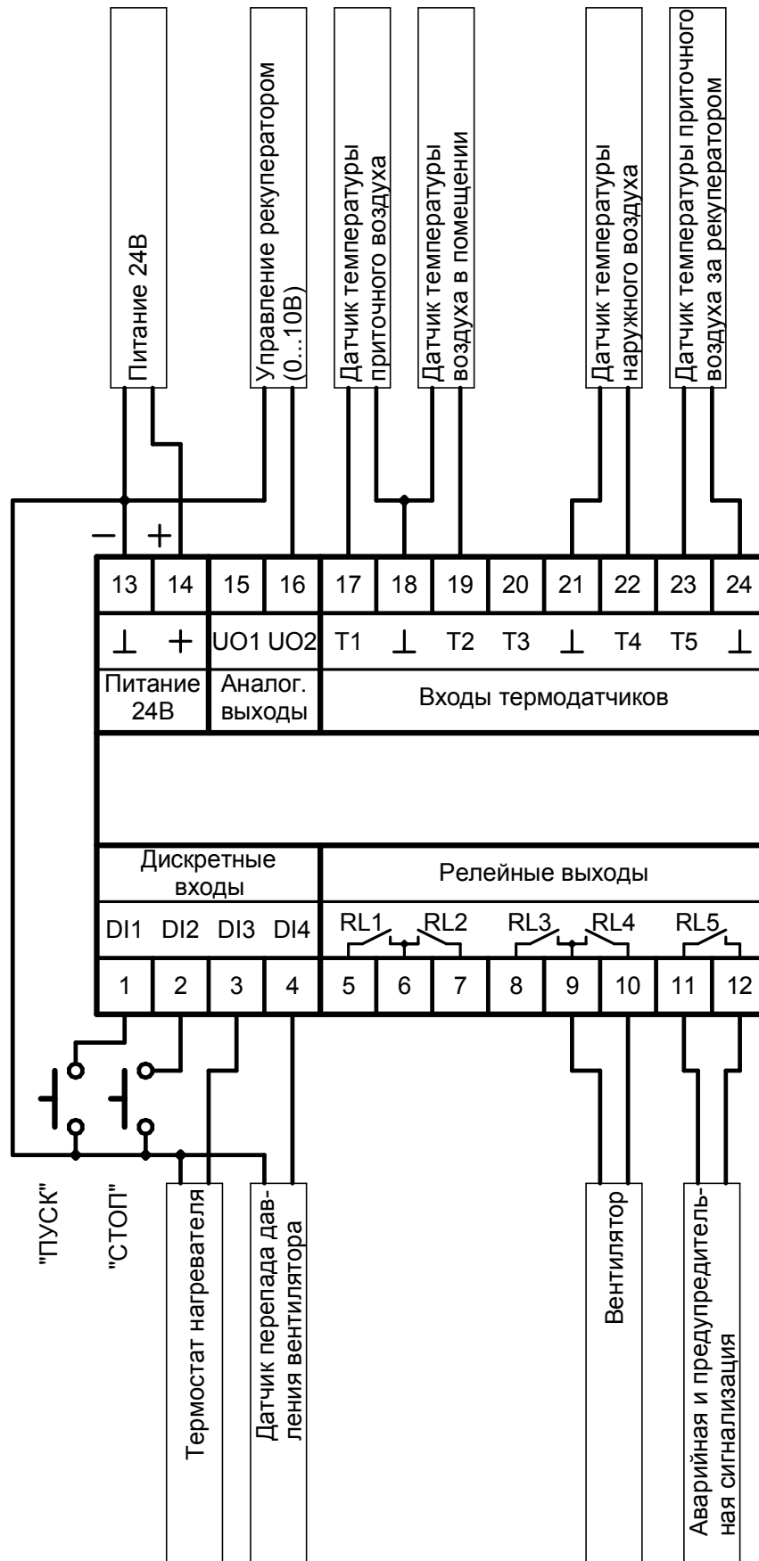
Рисунок 11. Подключение рекуператора.
