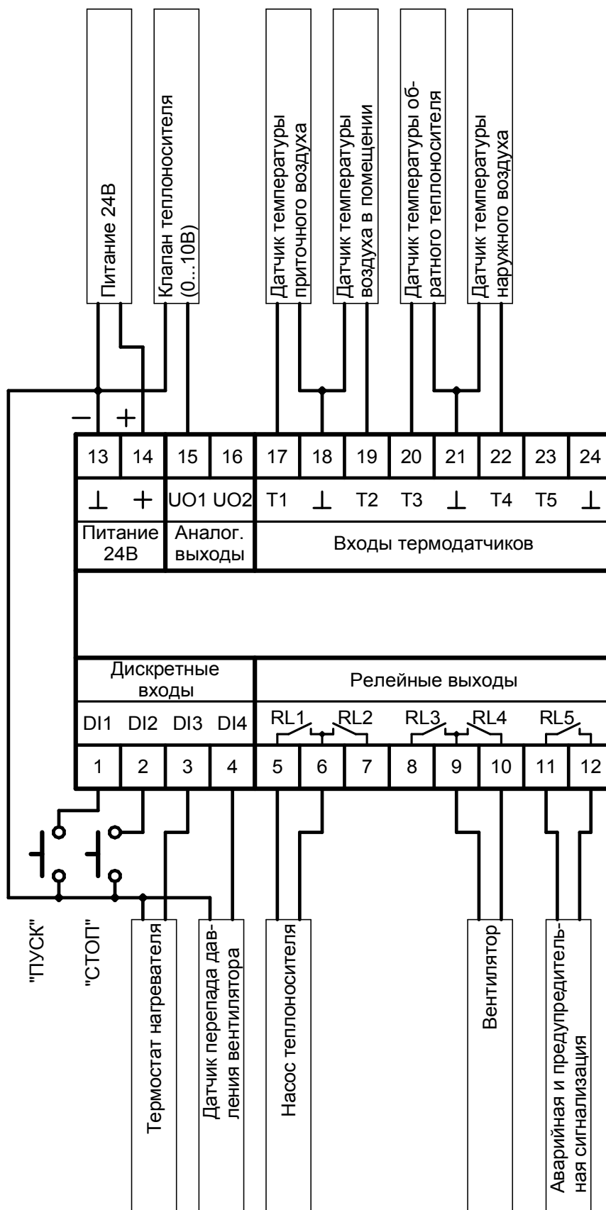
Рисунок 6. Подключение ВВН.
