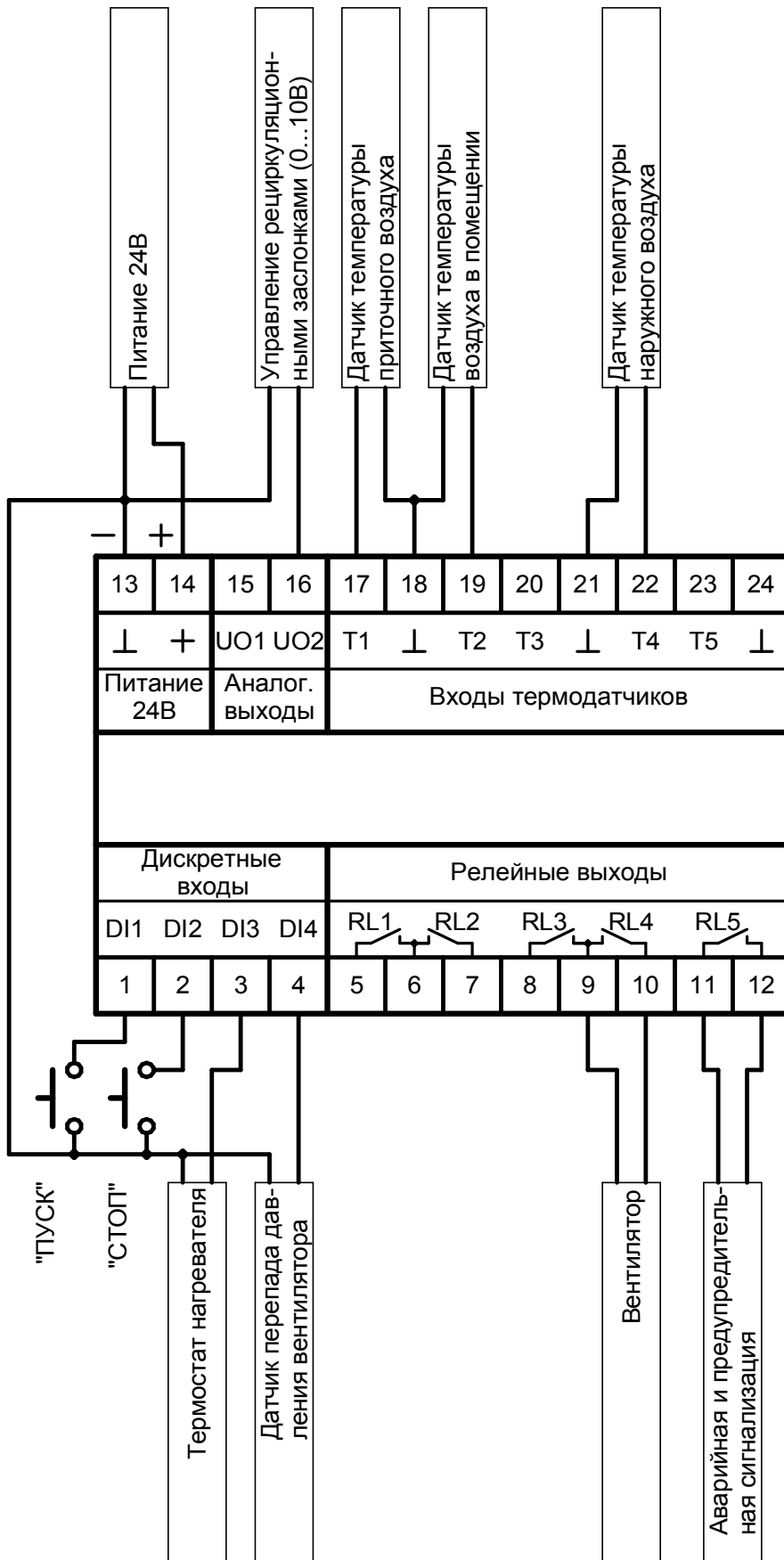
Рисунок 12. Подключение рециркуляционных заслонок.
