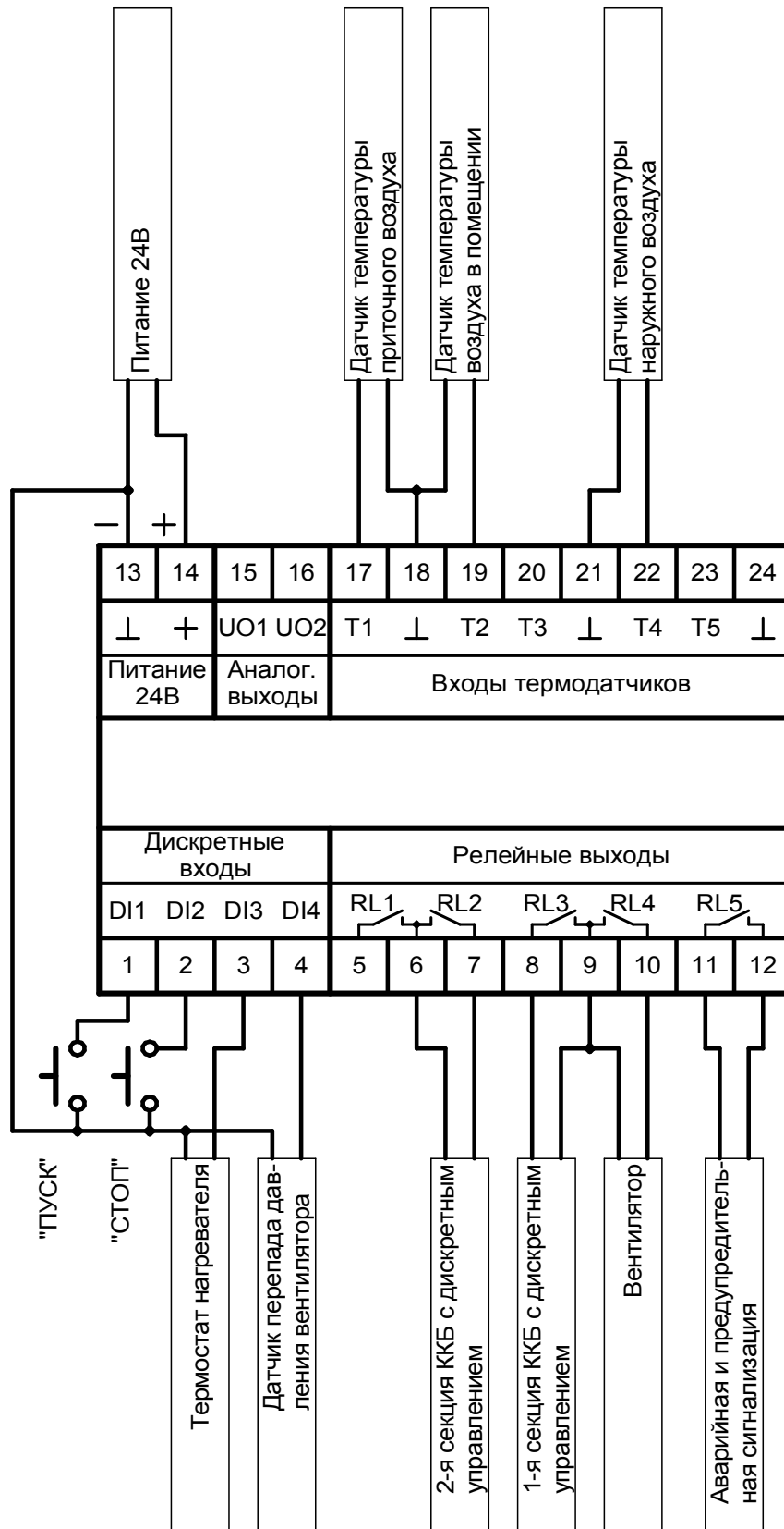
Рисунок 9. Подключение ККБ с дискретным управлением.
