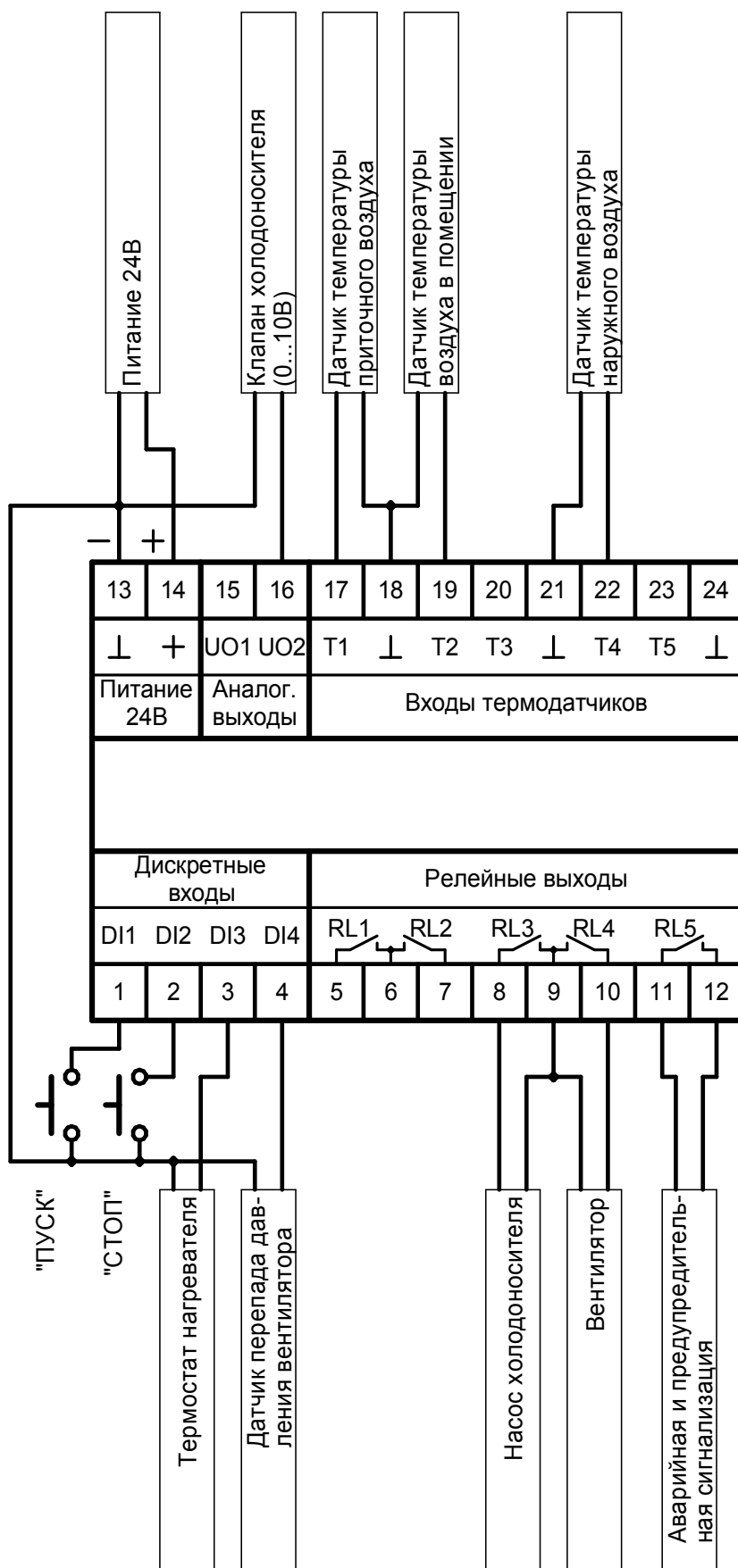
Рисунок 8. Подключение ВВО.
